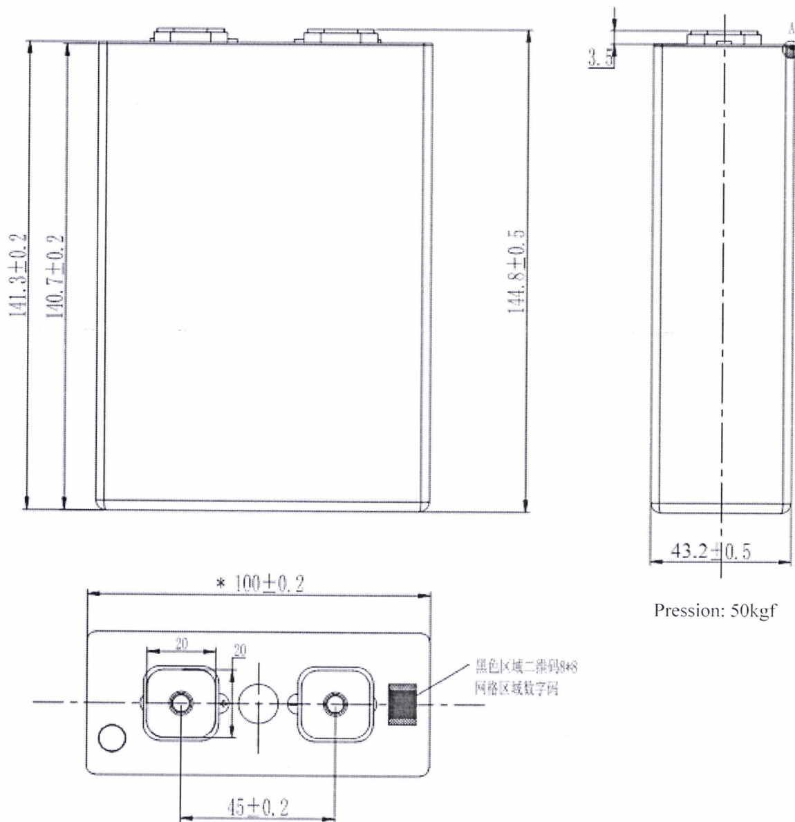
电芯整体尺寸
